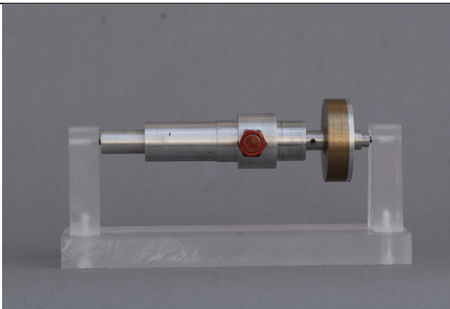
EC(H)O Auswuchtsystem Modell Welle
